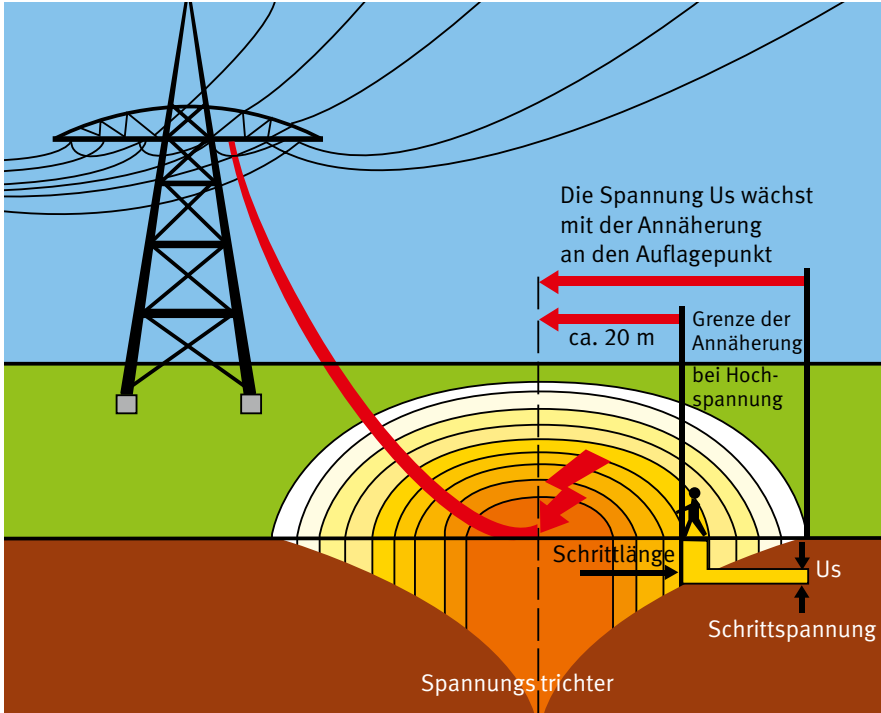
Spannungsrichter
